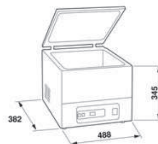
Dimensions D300
