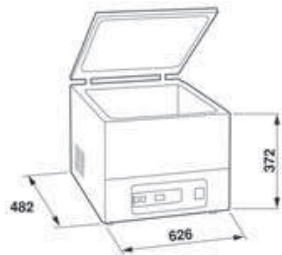
Dimensions D400
